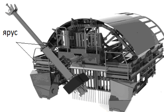
Рисунок 1. Концепт-проект однорычажного укладчика
